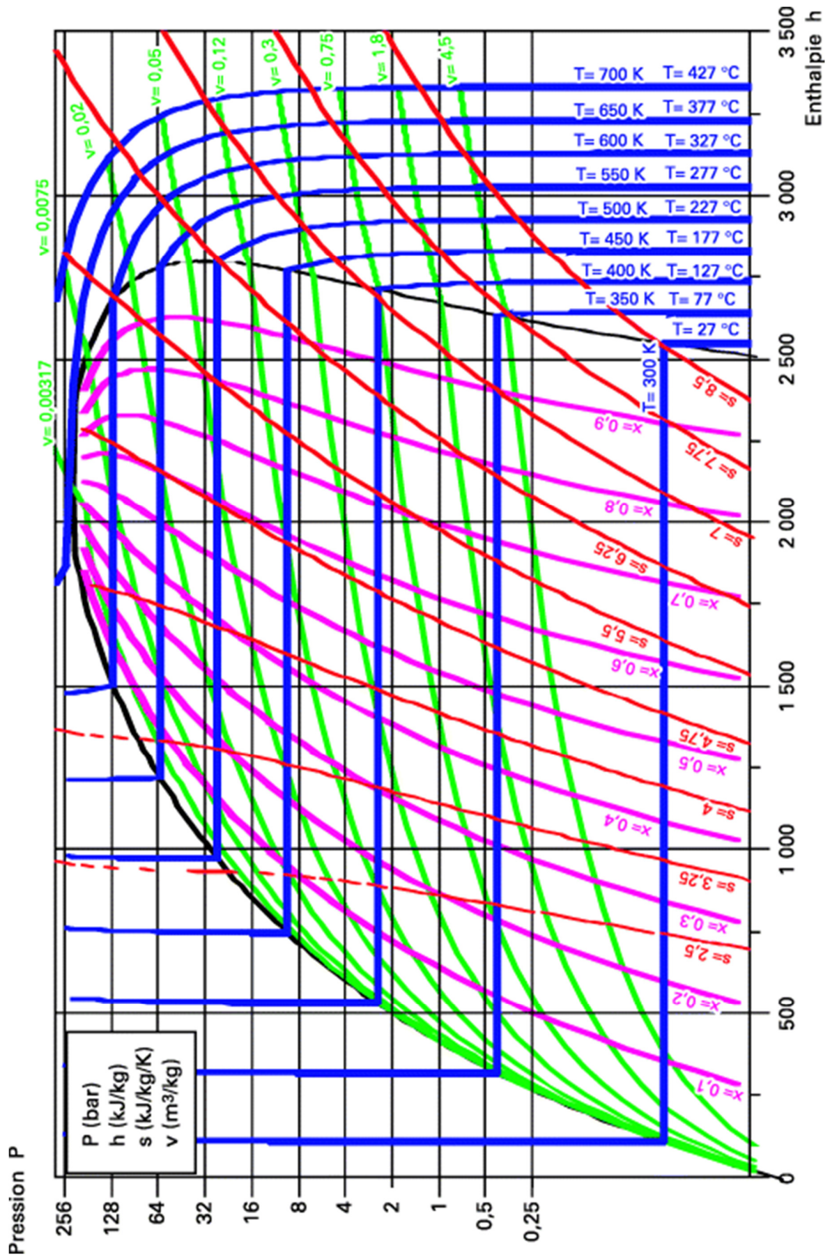
Diagramme (h, ln(P)) de l'eau
